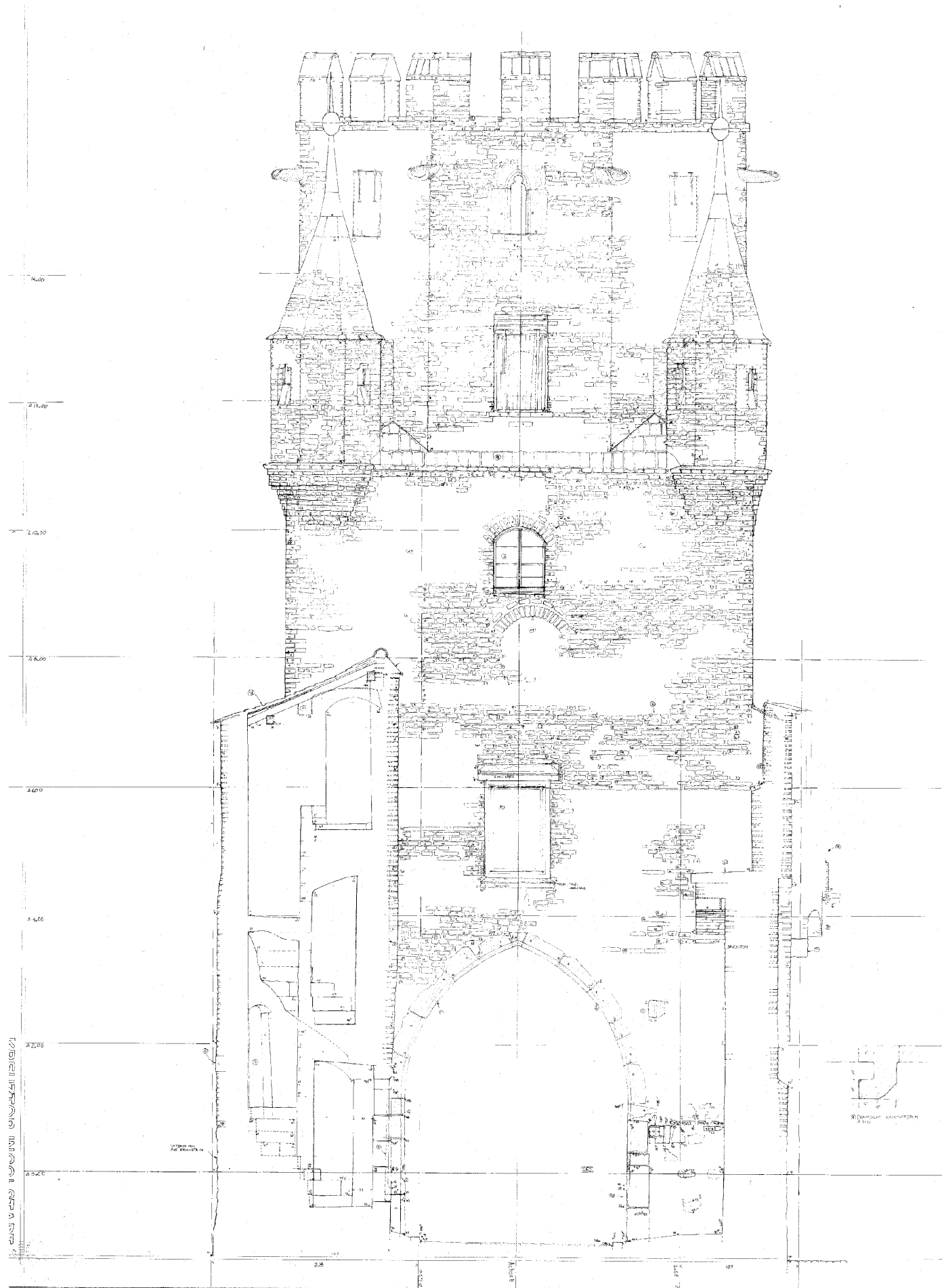
Kreuztor in Ingolstadt / Westansicht : Steingerechtes Handaufmass als Grundlage für eine Schadenskartierung, Bleistift auf Karton ( Original im M 1:25 )
